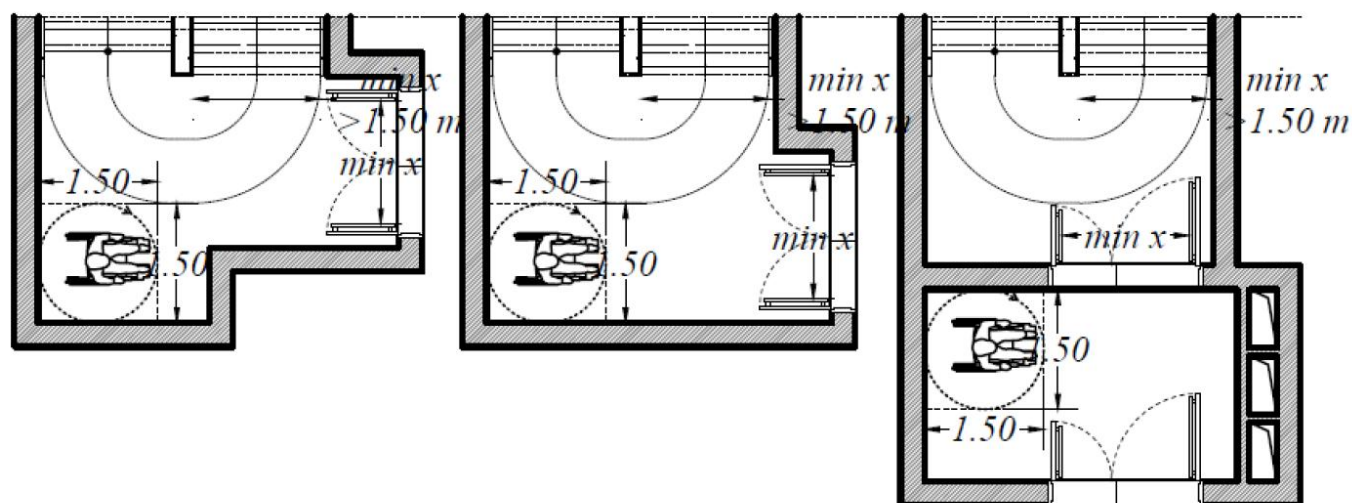
Figura 221 - Gabarit punct de staționare a persoanelor cu dizabilități - amplasare în scara de evacuare.
