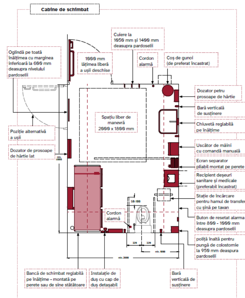
Fig. 29 Varianta 2 - plan grup sanitar cu pat de schimbat persoane adulte
