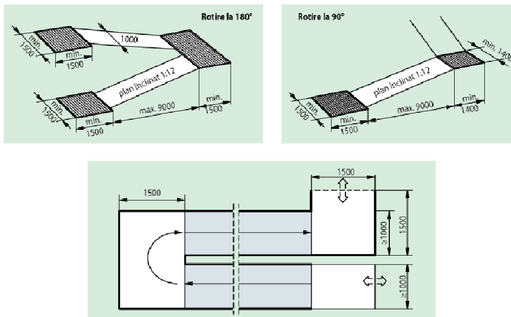
Fig. C.21 Planuri înclinate
